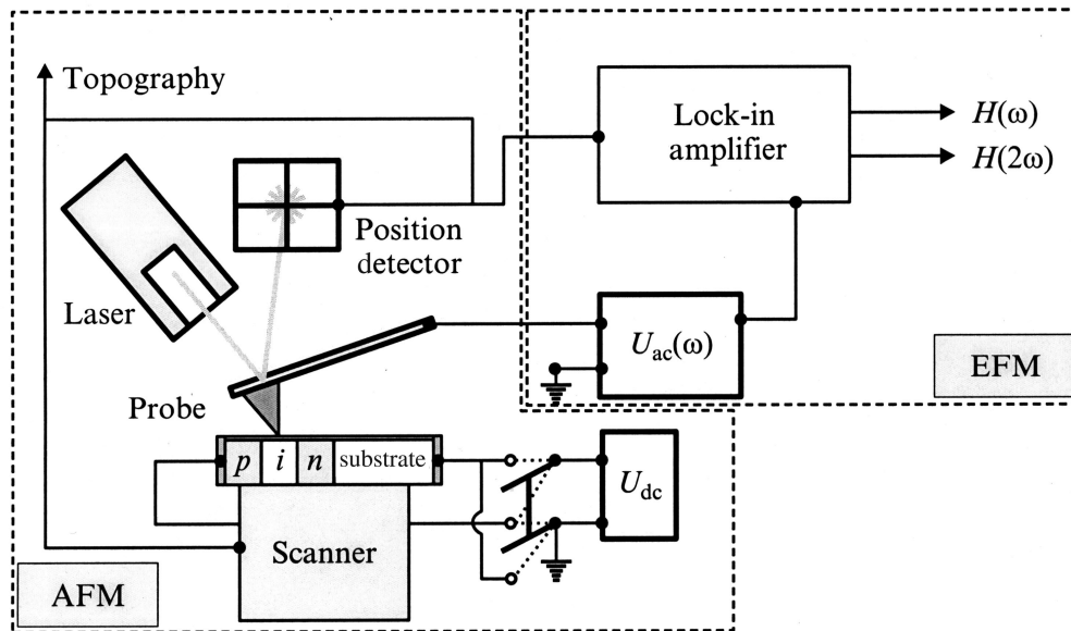
Рис. 1. Экспериментальная установка.
